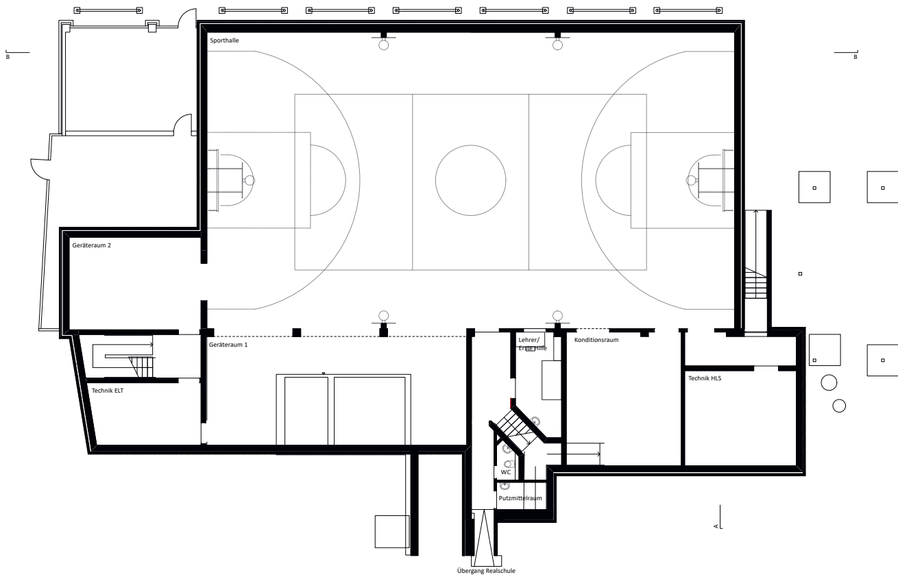
08 Grundriss Untergeschoss
